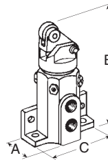
TASTROLLE (LEERRÜCKLAUF)
