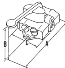
4/2-FEDERRÜCKHOLUNG
