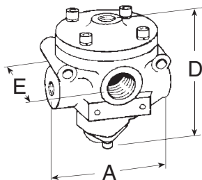
3/2-Wege-Sitzventile
