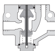
3/2 Normal geschlossen
